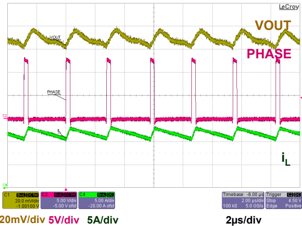
Fig. 12: CCM (I OUT = 12A) 2
